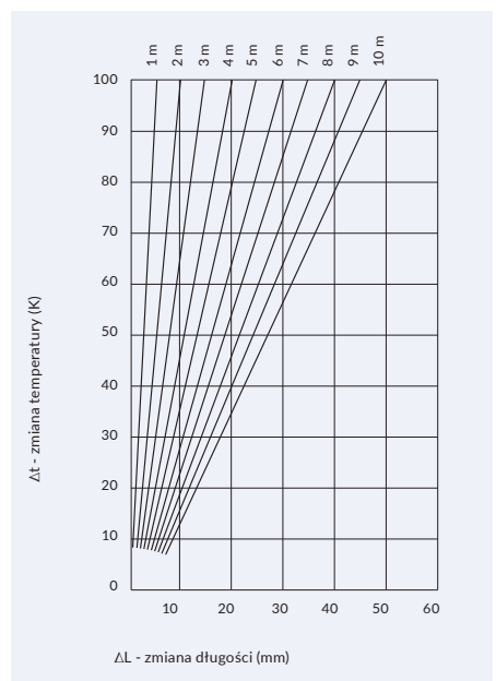
wykres 2. Rury Stabi \xi_t = 0,03 \text{ mm/m}^\circ\text{K}
