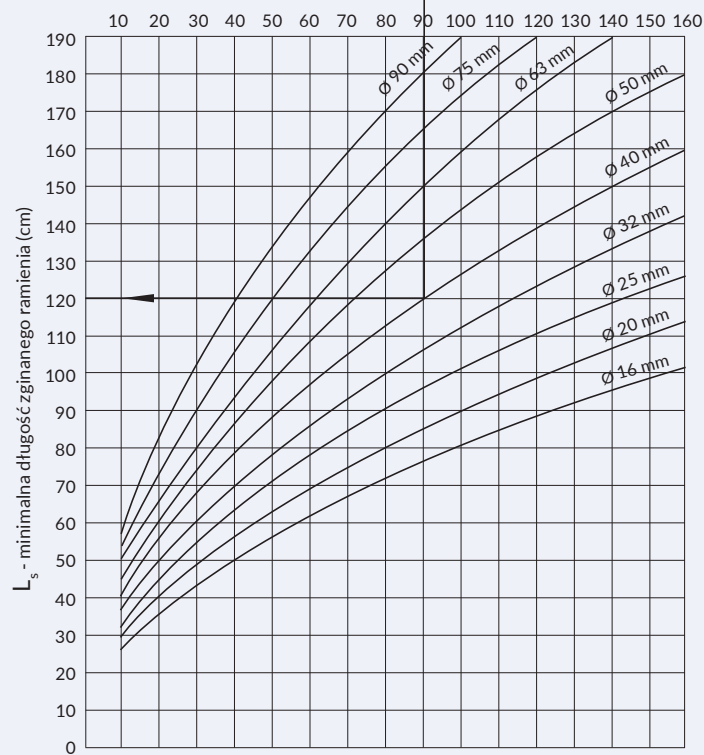
wykr. 5. i 6 układ wykresów do przybliżonego, graficznego określenia długości zginanego ramienia L_s .
